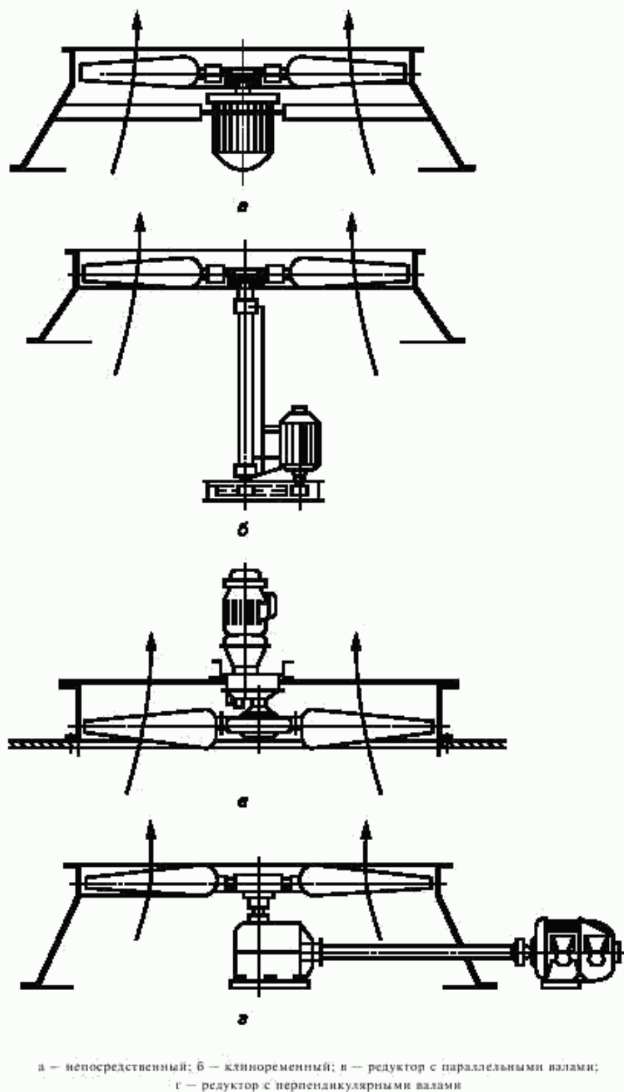
Рисунок 6 — Приводы аппаратов вытяжного вида
